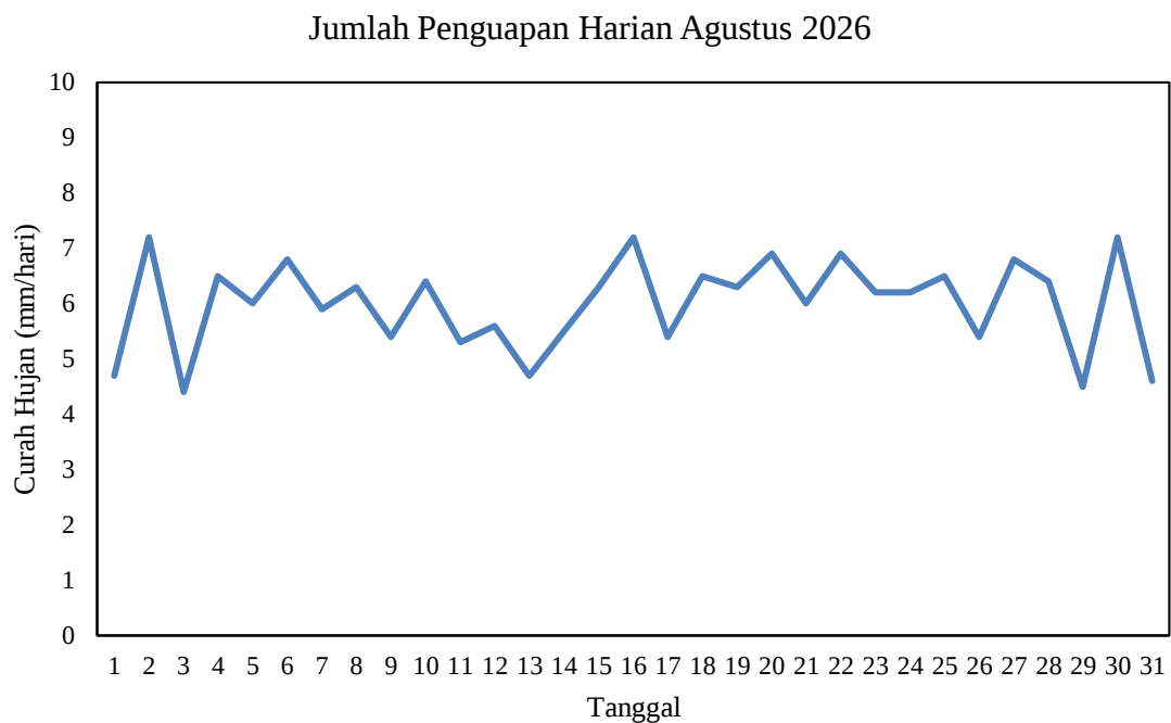
Gambar 2.8 Grafik Jumlah Penguapan Harian bulan Agustus 2026 di Stasiun Meteorologi Mali - Alor
