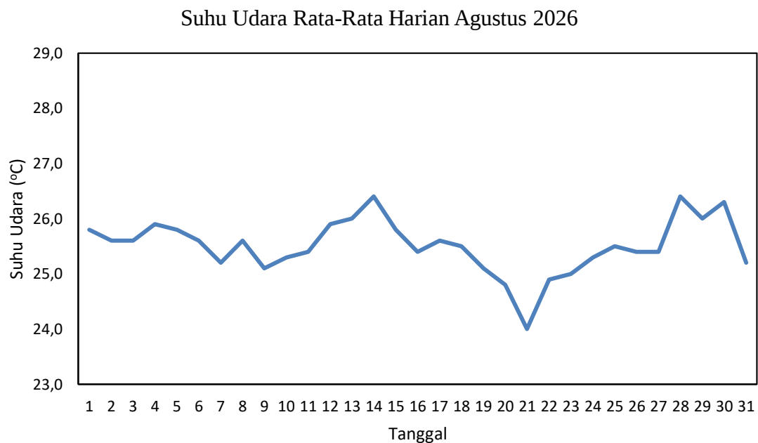
Gambar 2.1 Grafik Suhu Udara Rata-rata Harian Bulan Agustus 2026 di Stasiun Meteorologi Mali - Alor
