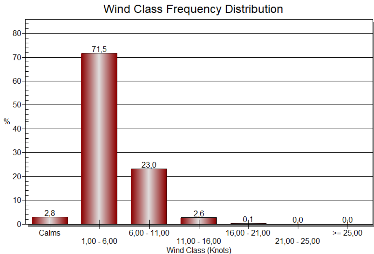
Gambar 2.10 Distribusi Frekuensi Angin Permukaan Bulan Agustus 2026 di Stasiun Meteorologi Mali - Alor
