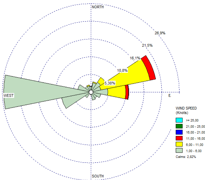
Gambar 2.9 Wind Rose Angin Permukaan Bulan Agustus 2026 di Stasiun Meteorologi Mali - Alor
