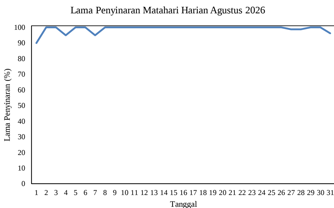
Gambar 2.7 Grafik Lama Penyinaran Matahari Harian bulan Agustus 2026 di Stasiun Meteorologi Mali - Alor
