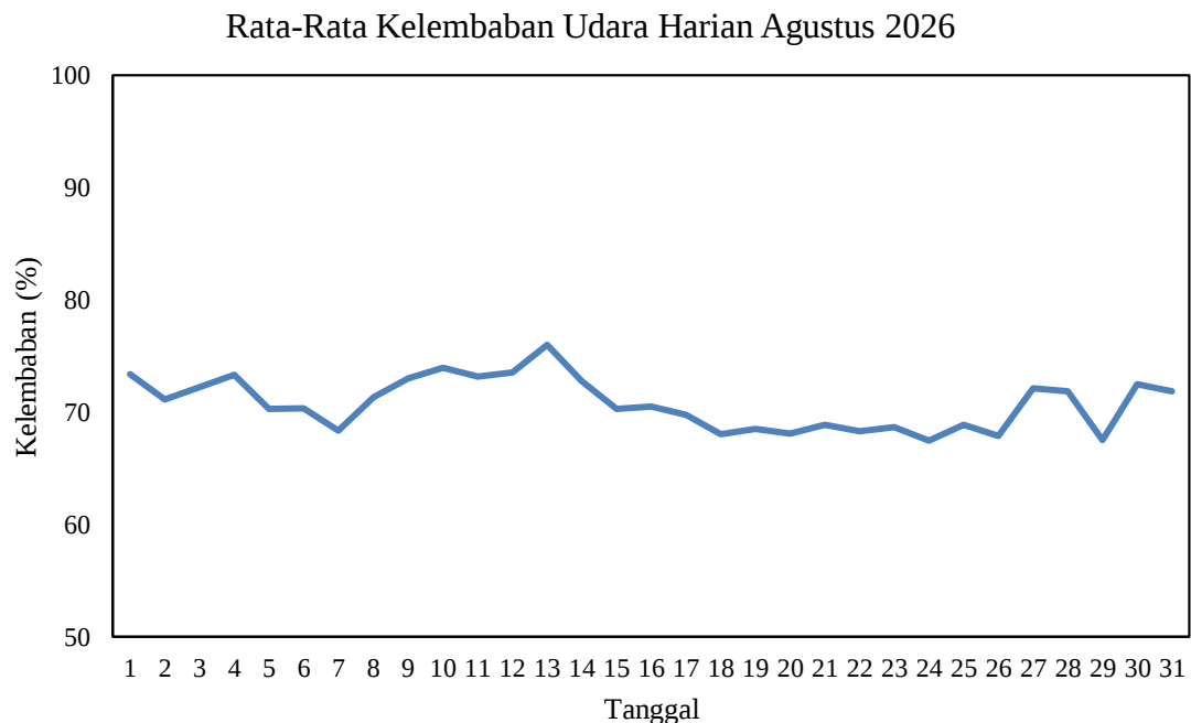
Gambar 2.5 Grafik Rata-rata Kelembaban Udara Harian Agustus 2026 di Stasiun Meteorologi Mali - Alor
