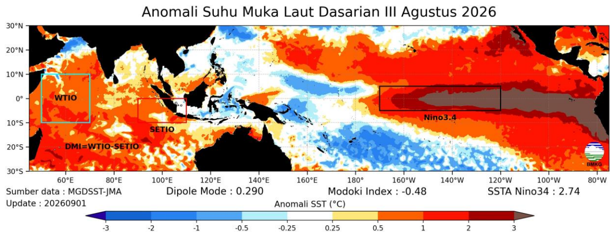
Gambar 3.2 Anomali Suhu Muka Laut di sekitar wilayah Indonesia pada Dasarian III bulan Agustus 2026
