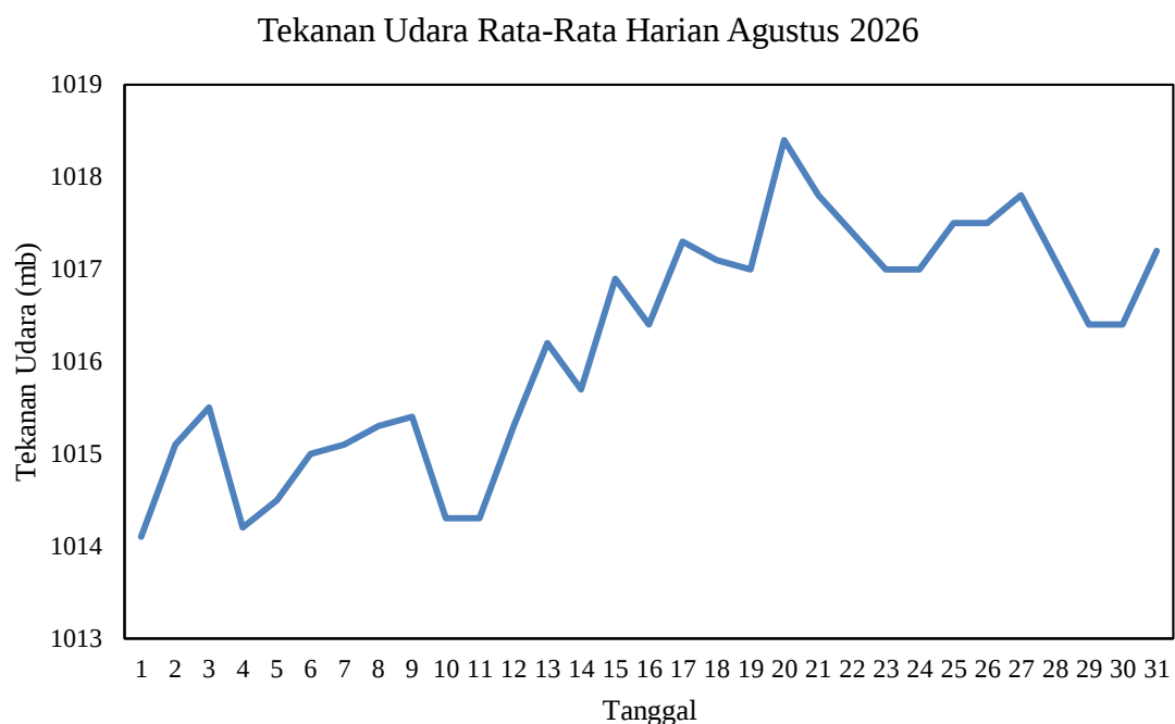
Gambar 2.6 Grafik Tekanan Udara Rata-rata Harian bulan Agustus 2026 di Stasiun Meteorologi Mali - Alor
