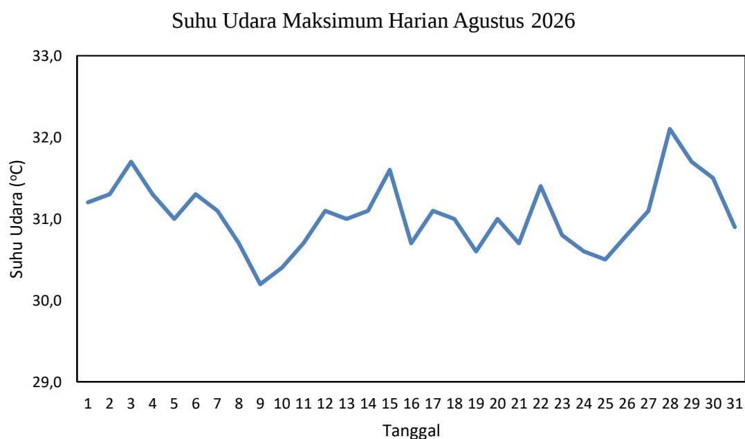
Gambar 2.2 Grafik Suhu Udara Maksimum Agustus 2026 di Stasiun Meteorologi Mali - Alor
