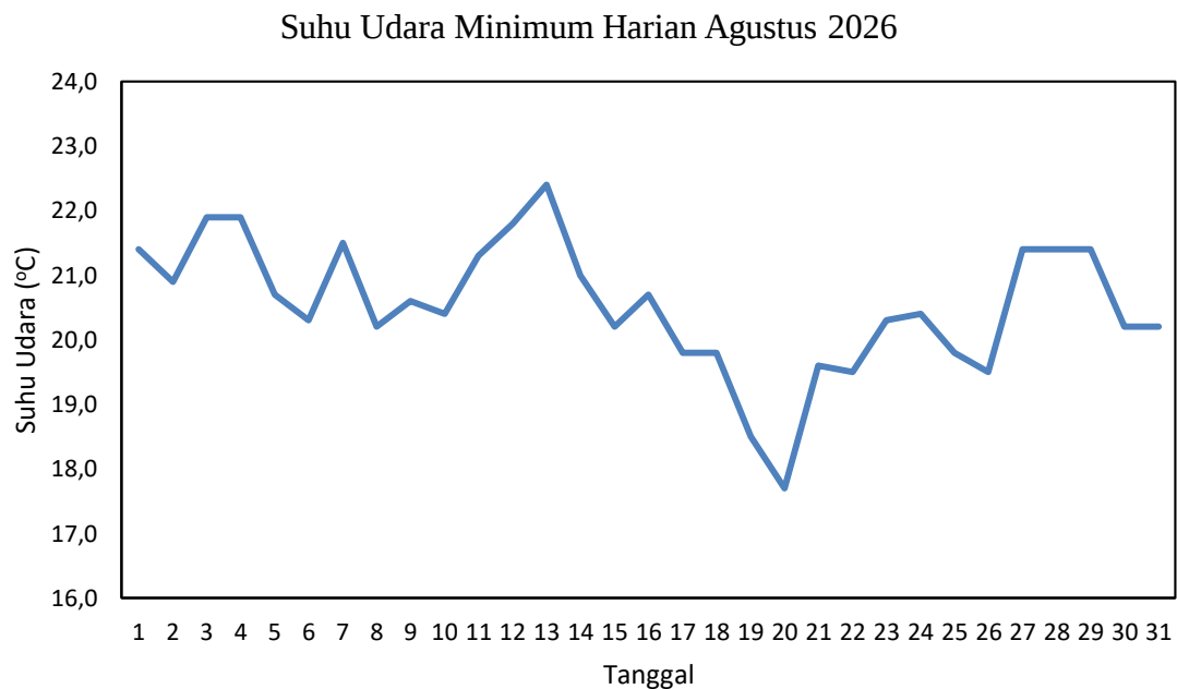
Gambar 2.3 Grafik Suhu Udara Minimum Agustus 2026 di Stasiun Meteorologi Mali - Alor
