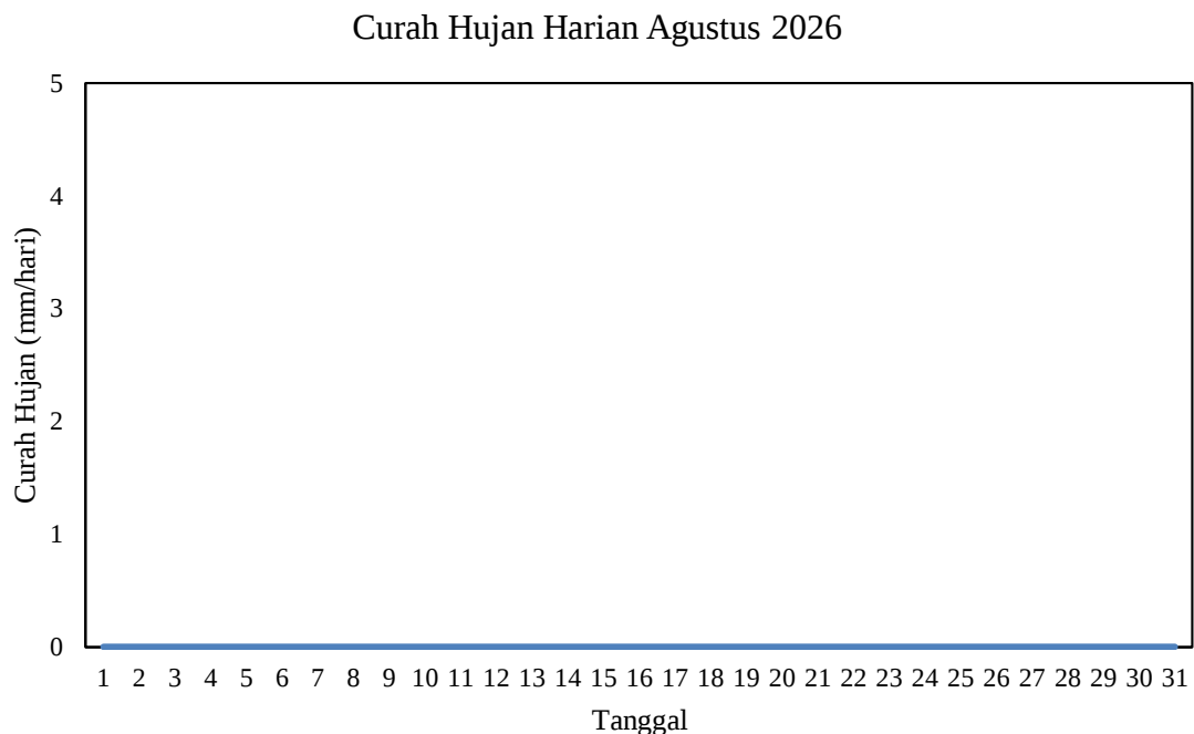
Gambar 2.4 Grafik Curah Hujan Harian Agustus 2026 di Stasiun Meteorologi Mali - Alor
